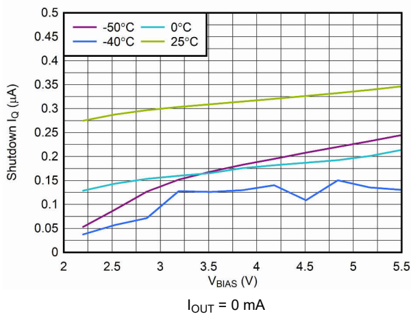
Figure 6-9. V_{\text{BIAS}} Shutdown I_{\text{Q}} vs V_{\text{BIAS}}
